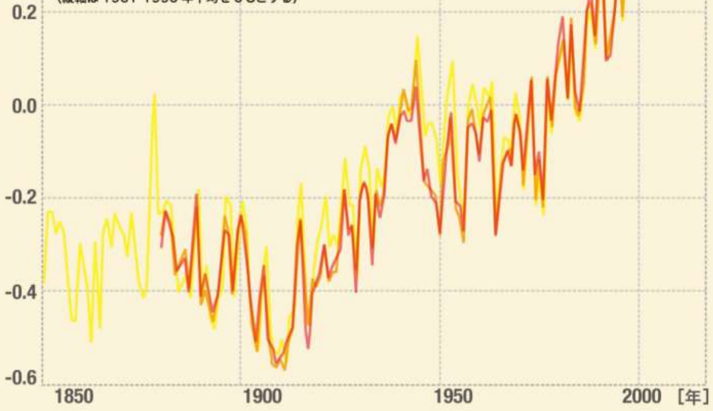
世界の地上気温の経年変化(年平均) 出典) IPCC第5次評価報告書 WGI Figure SPM.1 ※偏差の基準は 1961-1990 年平均 (縦軸は 1961-1990 年平均を 0°Cとする)
